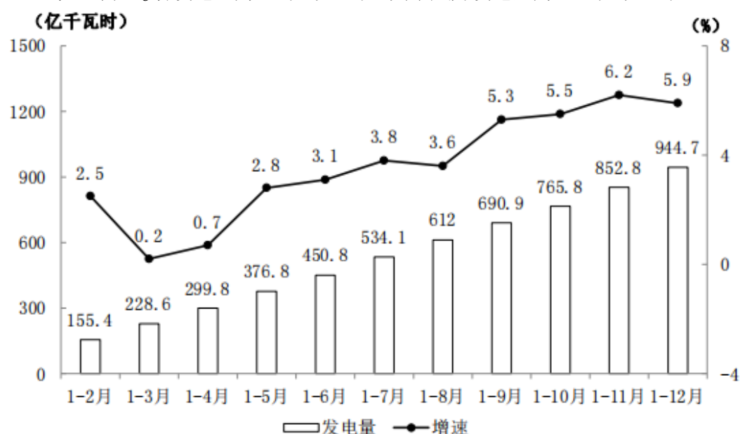
图1 2020年2-12月J省累计发电量及同比增速
