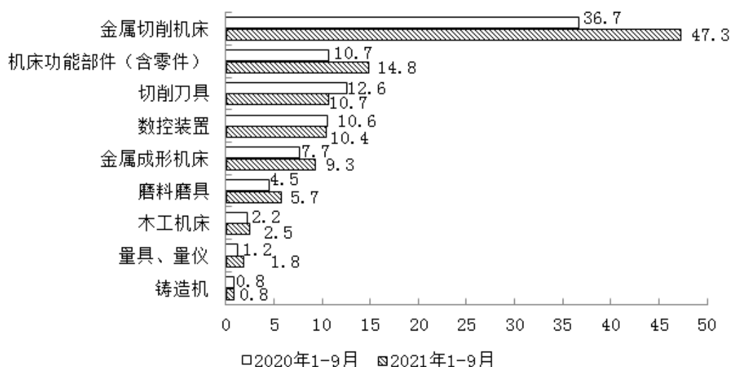
图2 我国机床工具产品累计出口情况（亿美元）
