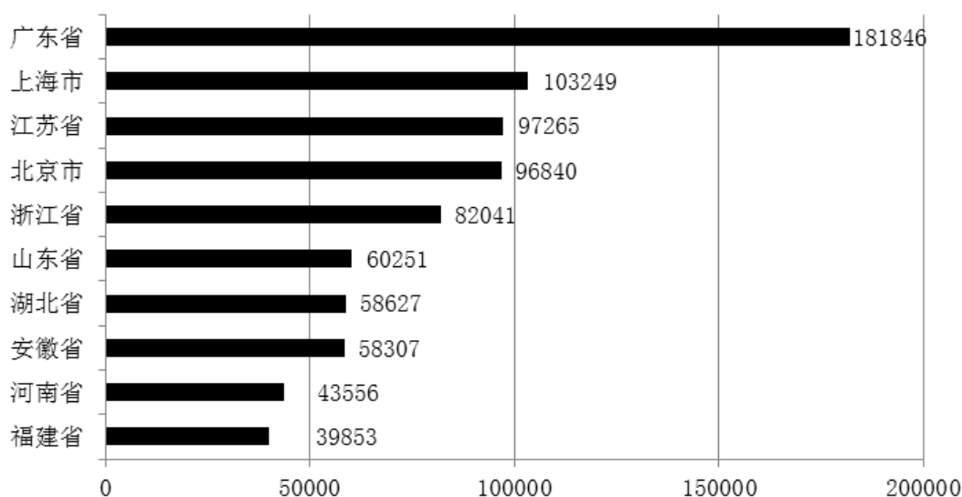
图2:2021年全国部分省级行政区公共充电桩数量TOP10（单位：台）
