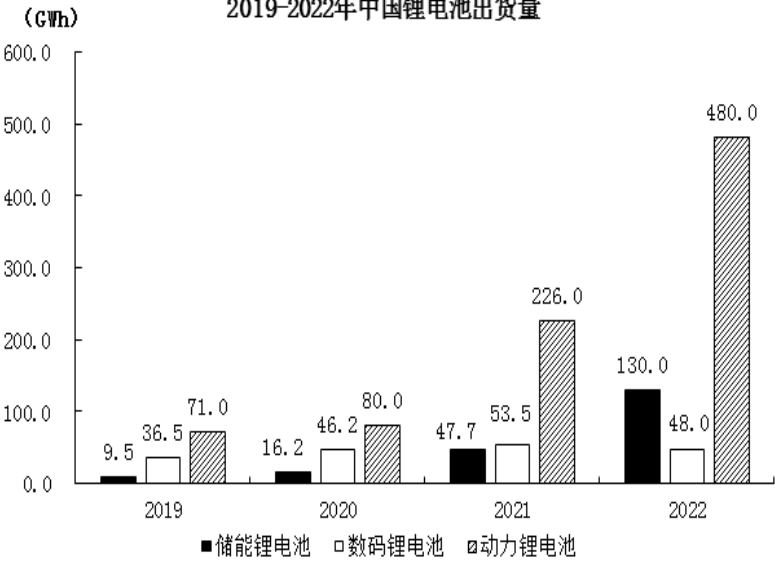
2019—2022年中国锂电池出货量
